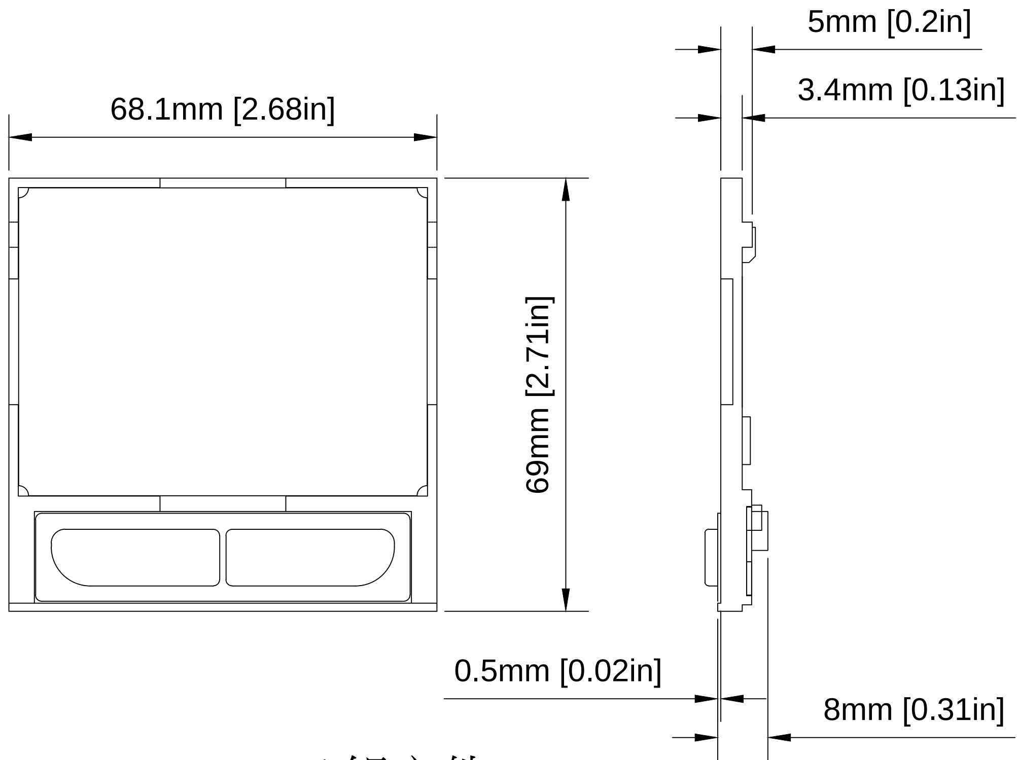
Mouse Pad 組立件
